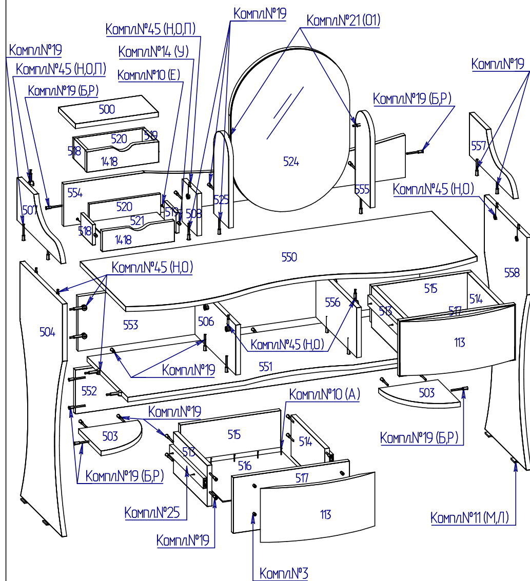
Крепление дна ящика (комплект №10)
